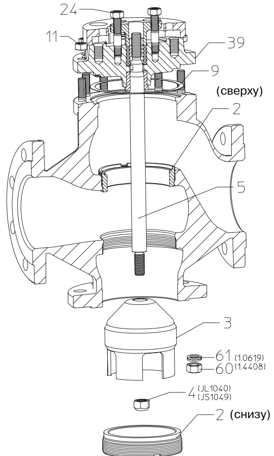
Рис. 21: BR450 DN125v-150v со смешительным затвором
