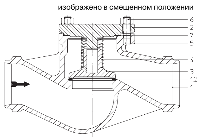
Рис. 4: Обратный клапан (предохранитель обратного потока) - DG SE (1.0619+N)
